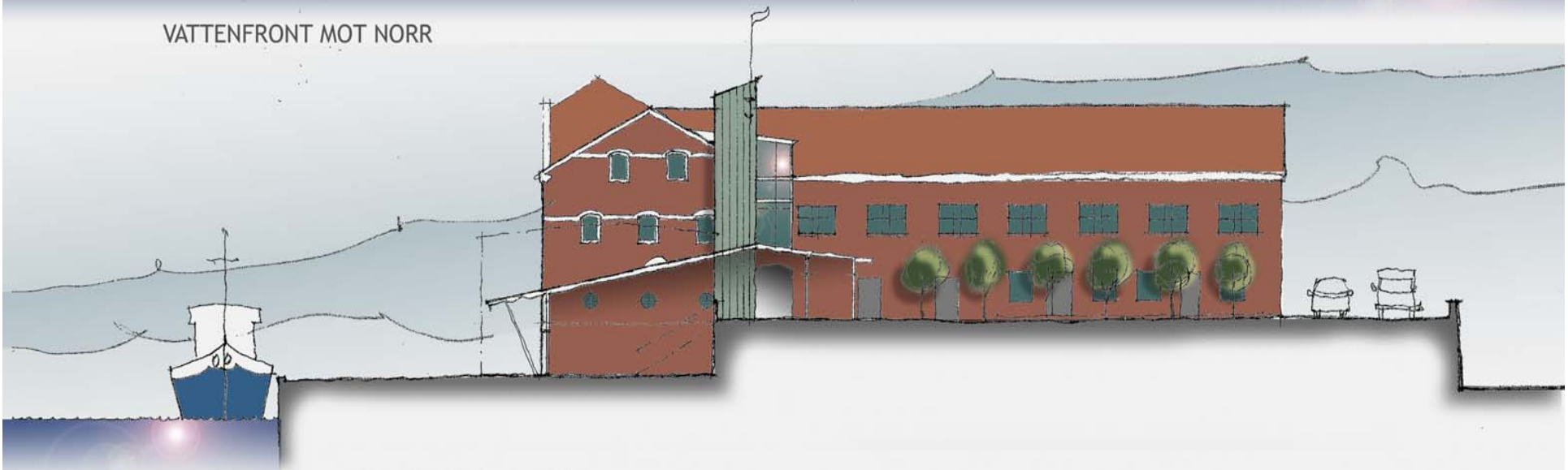
SEKTION KAJ - INOMHUSTORG - ENTRÉ
