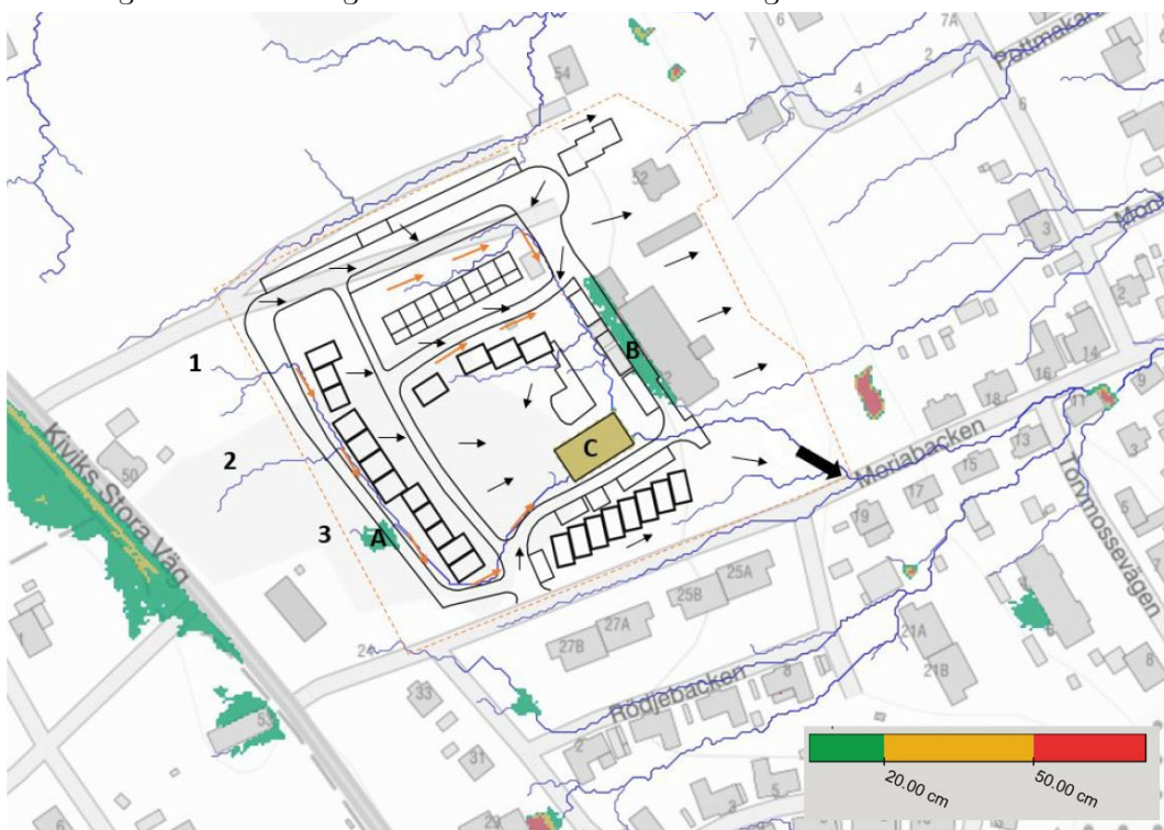
Figur 5 – Översiktligt förslag för skyfallshantering. Flödesvägar redovisas i blått, orange pilar redovisar rinnvägar i dräneringsstråken, svarta pilar redovisar den yttliga avrinningen. Vattendjup i lågpunkter enligt teckenförklaringen.
