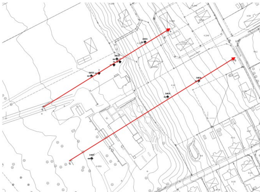
Figur 1 Valda sektioner för stabilitetsberäkningar
